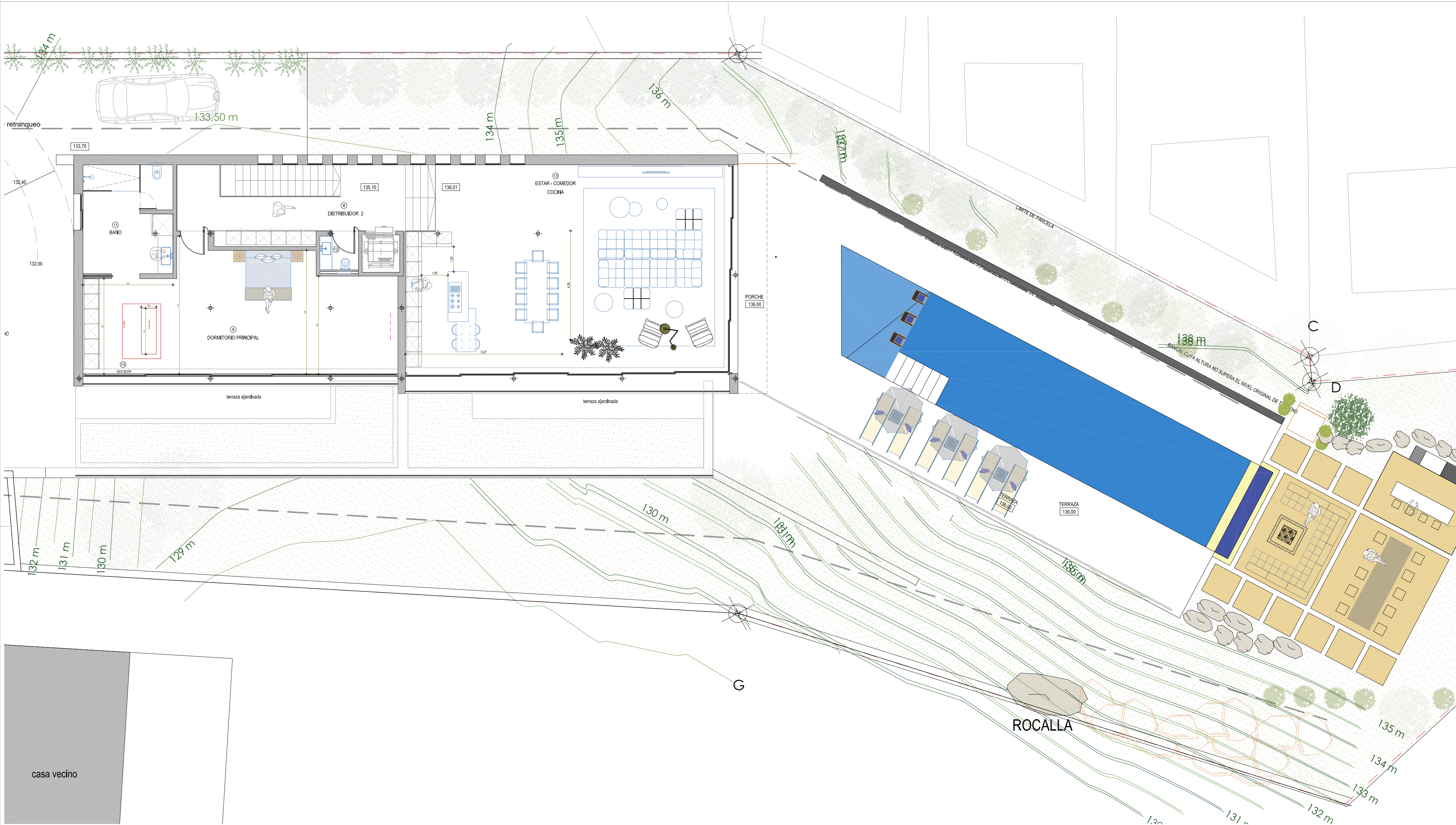
PLANTA PISO VIVIENDA Y TERRAZA CON PISCINA ESC: 1/100
